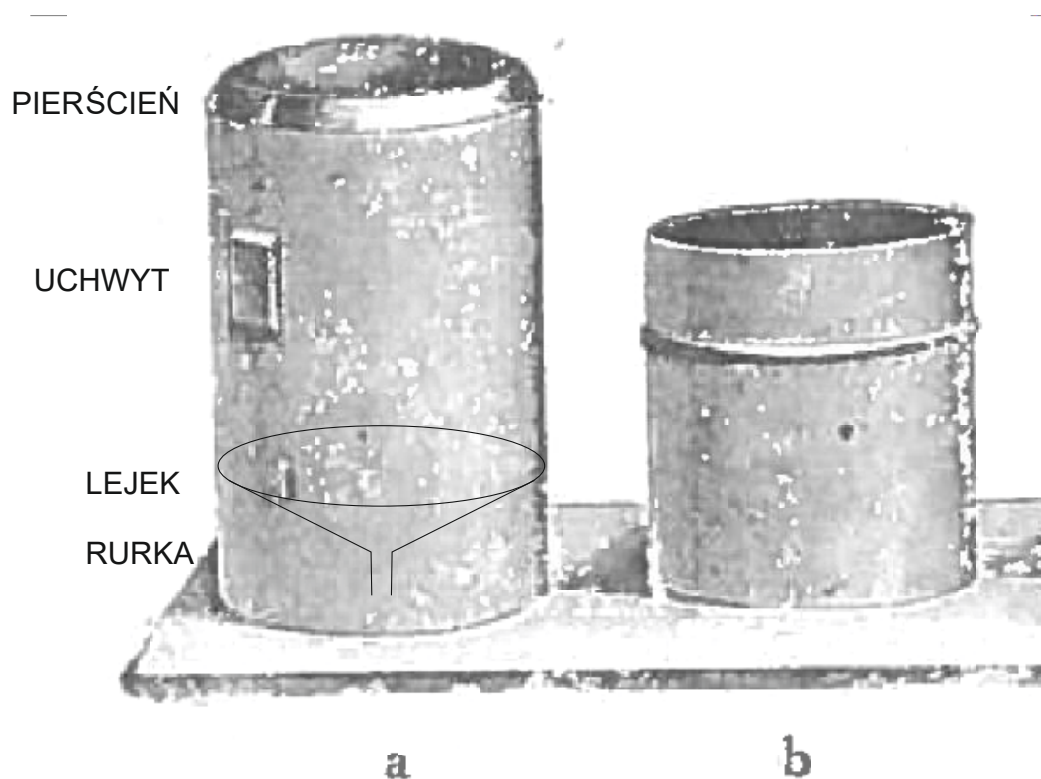
Rys 1b. Schematyczny rysunek deszczomierza Hellmanan a) odbiornika (wraz z zaznaczeniem budowy wewnętrznej), b) podstawy deszczomierza Hellmanna
