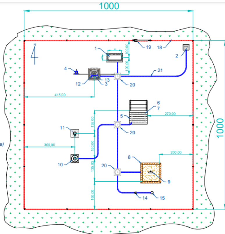
Rysunek 1 Schemat stacji klimatologicznej
