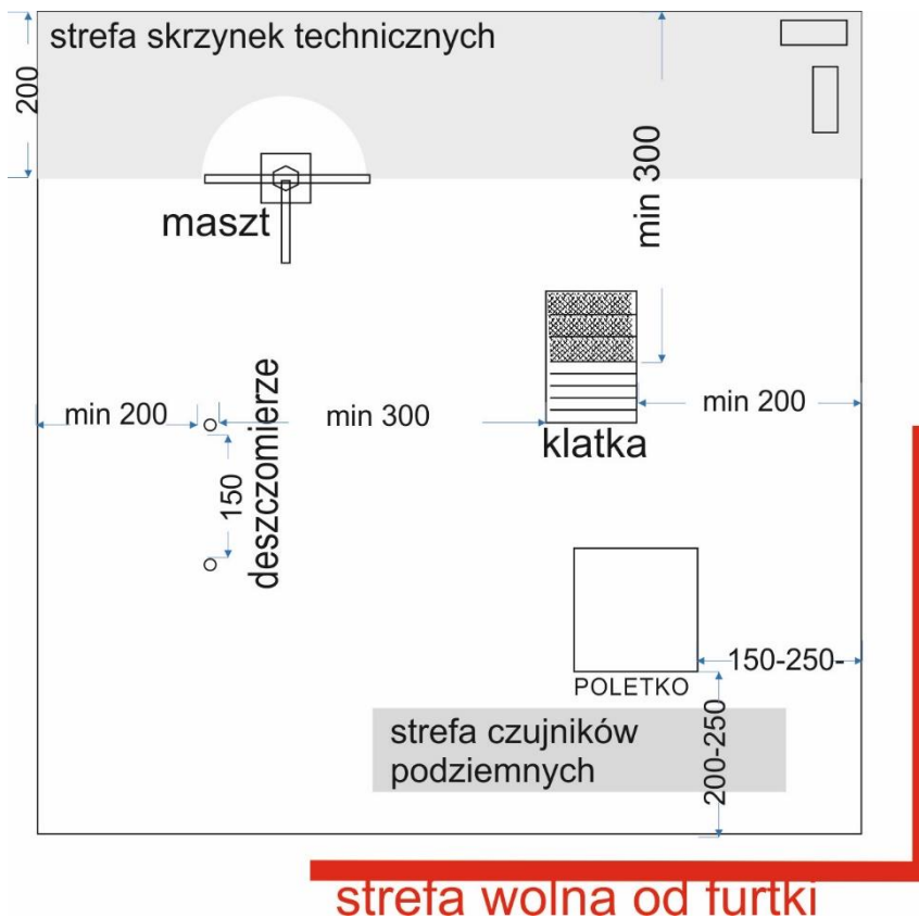
Rysunek 2 Ogródek stacji klimatologicznej z zaznaczonymi strefami w których powinny być umieszczone przyrządy
