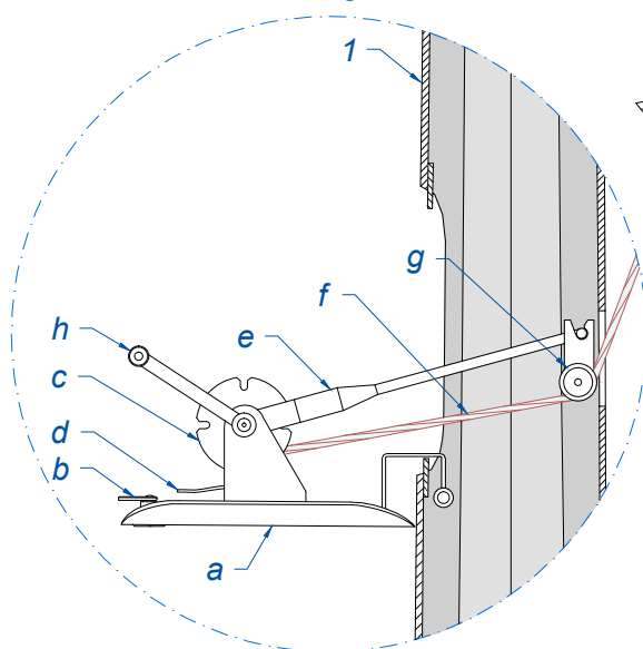
Szczegół A1
