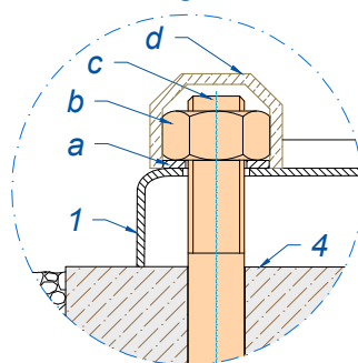
Szczegół A2
